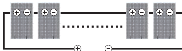
Collegamento in serie per ottenere valori di tensione superiori
