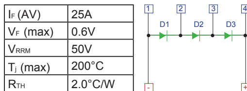
Specifiche e configurazione dei diodi
