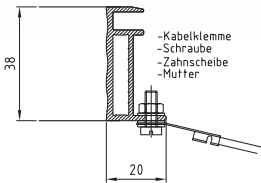
„Erdanschluß“
